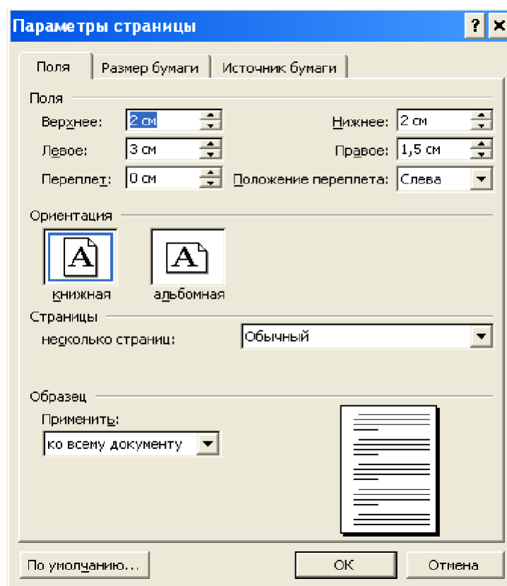
Рис. 6.1. Параметры страницы
