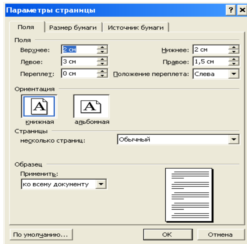
Рис. 3.1. Параметры страницы
