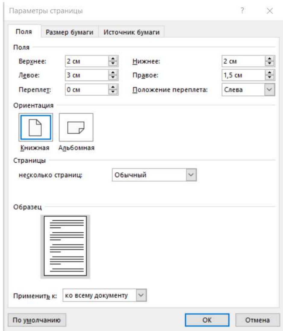
Рис. 5.1. Параметры страницы
