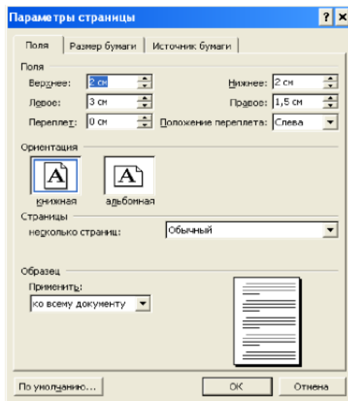
Рис. 4.1. Параметры страницы
