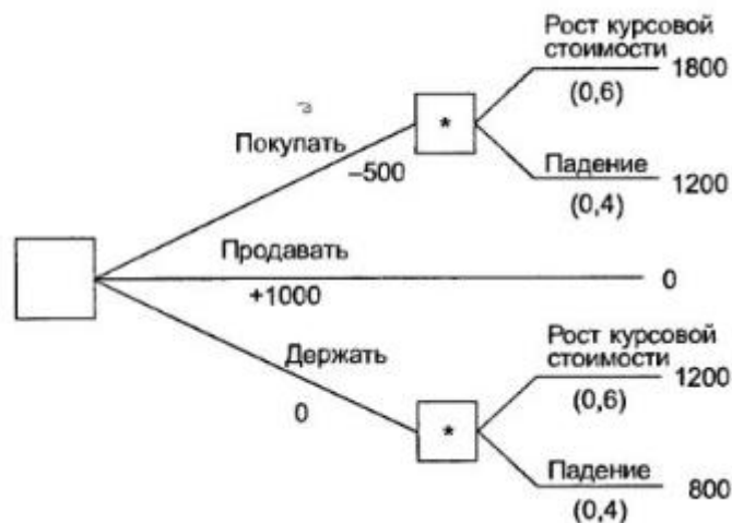
Рис. 2. Дерево решений
