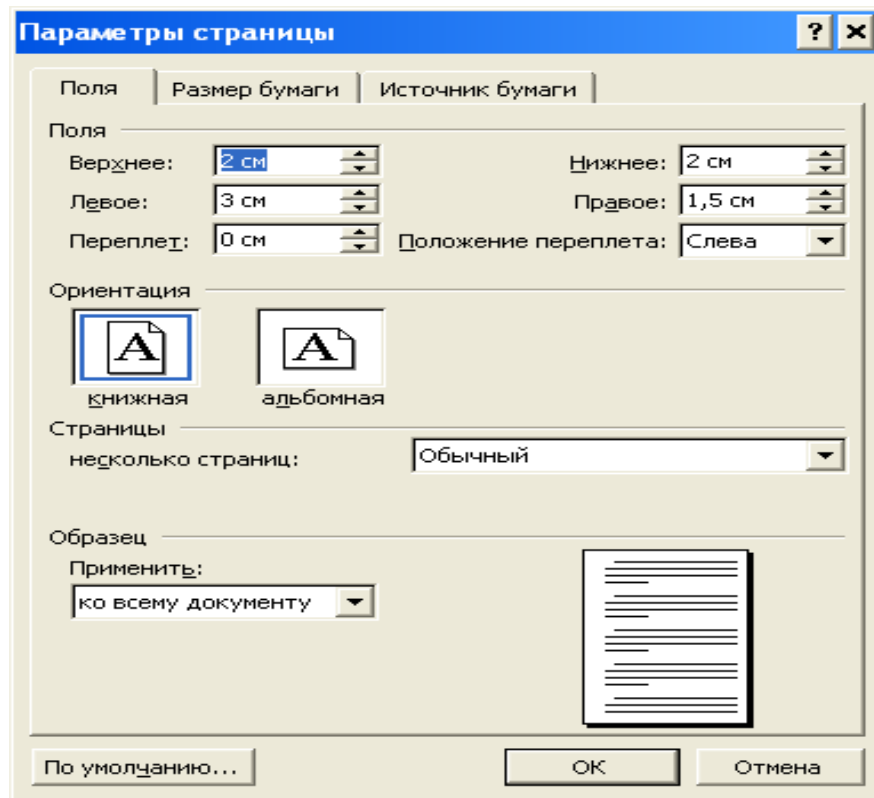
Рис. 4.1. Параметры страницы
