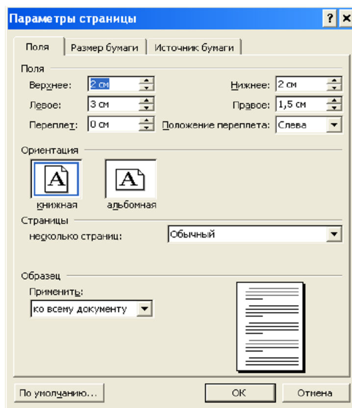
Рис. 5.1. Параметры страницы
