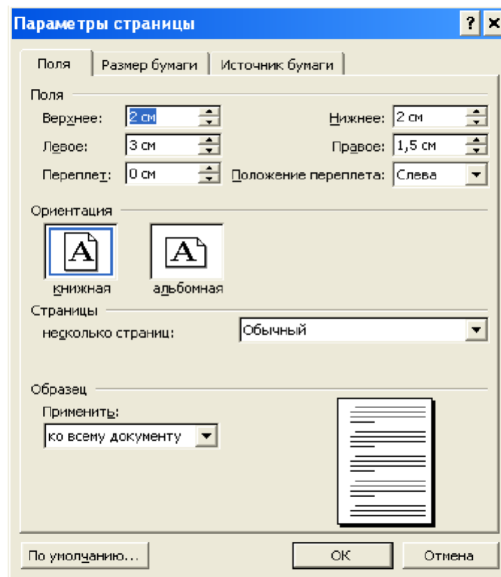
Рис. 5.1. Параметры страницы
