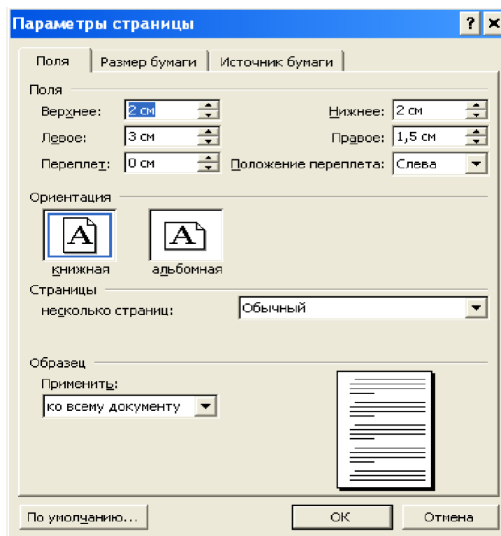
Рис. 8.1. Параметры страницы
