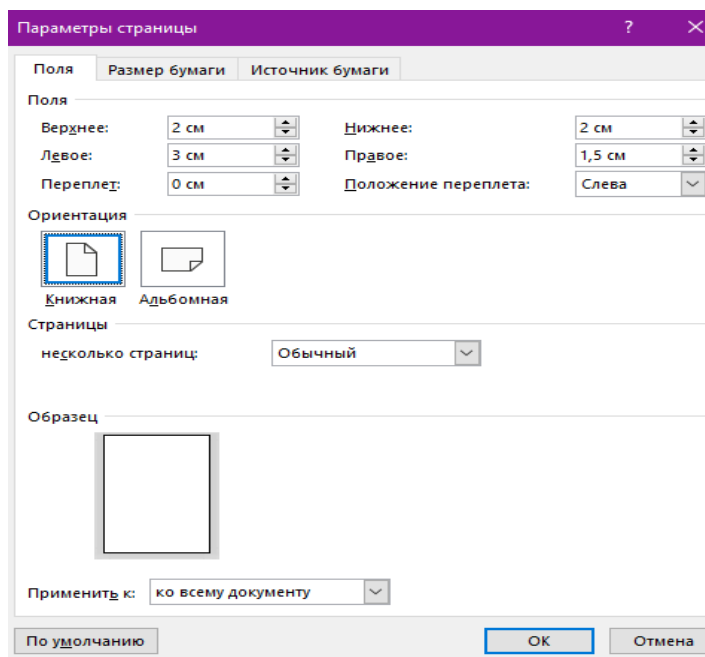
Рис. 8.2. Параметры страницы
