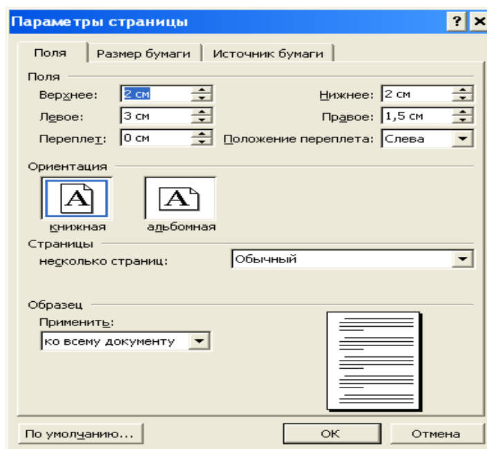
Рис. 4.1. Параметры страницы
