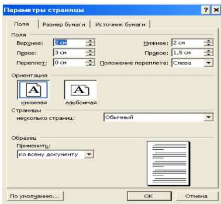
Рис. 5.1. Параметры страницы
