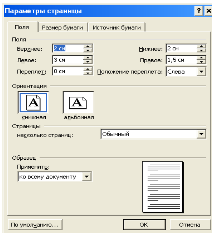
Рис. 7.1. Параметры страницы
