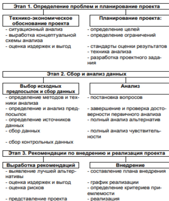
Рис. 4. Этапы проектирования и планирования цепей поставок
